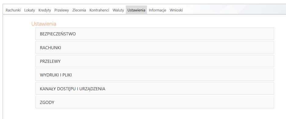
Rys. 43 Okno „Ustawienia”
